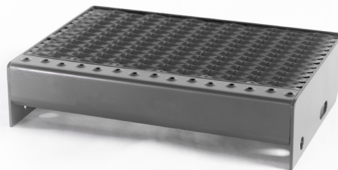
Stupeň s všesměrově protiskluzovým tahokovem Safe 45x13,4/5mm
